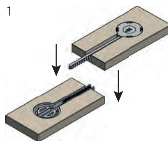
Схема монтажа №2
